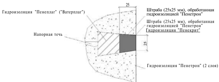
Узел примыкания при строительстве
