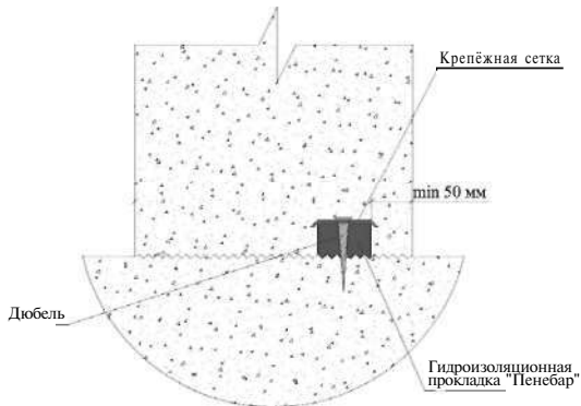
Узел примыкания при строительстве
